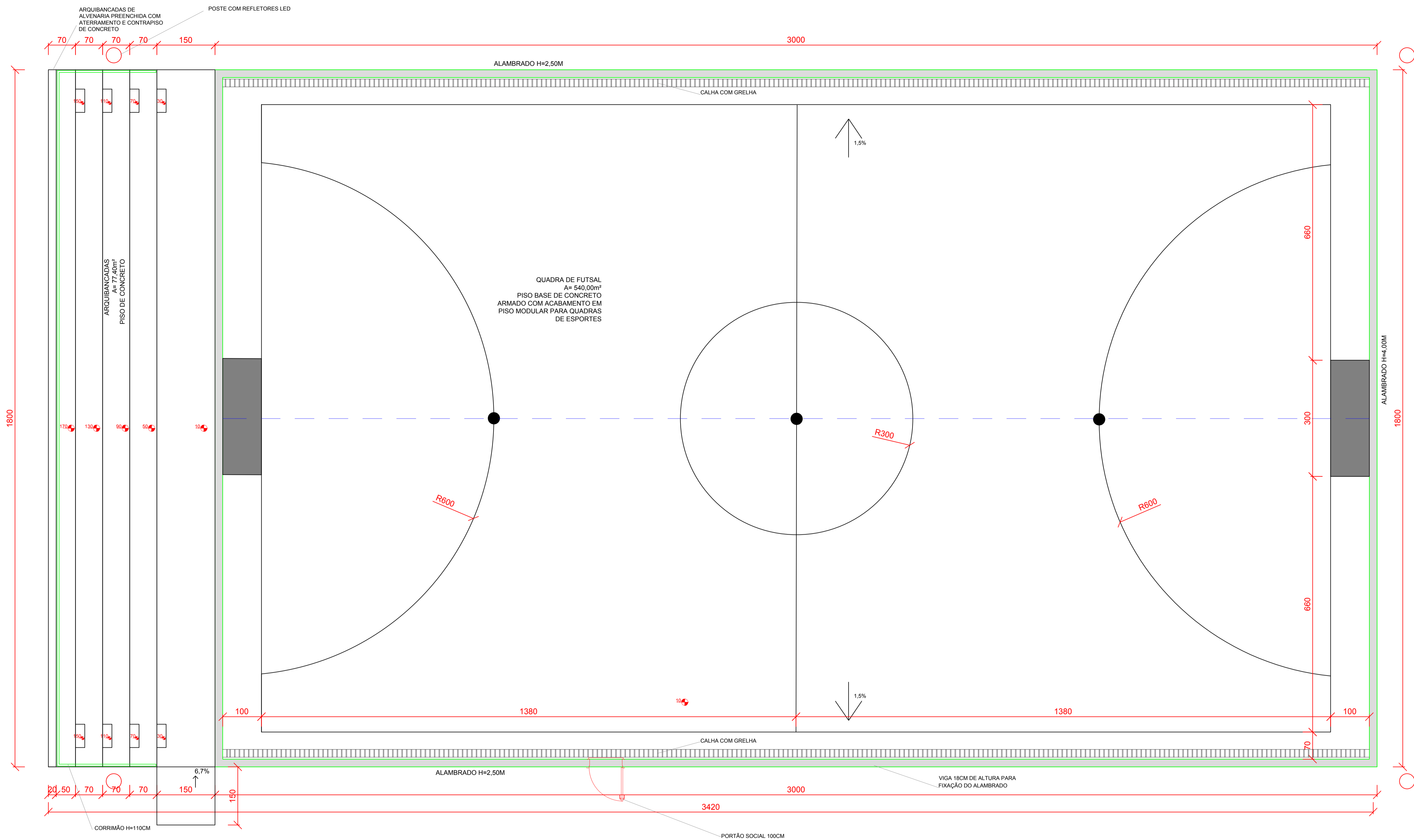
— ENG PLANTA BAIXA QUADRA FUTSAL - TAMANHO NÃO OFICIAL ESCALA - 1/50
