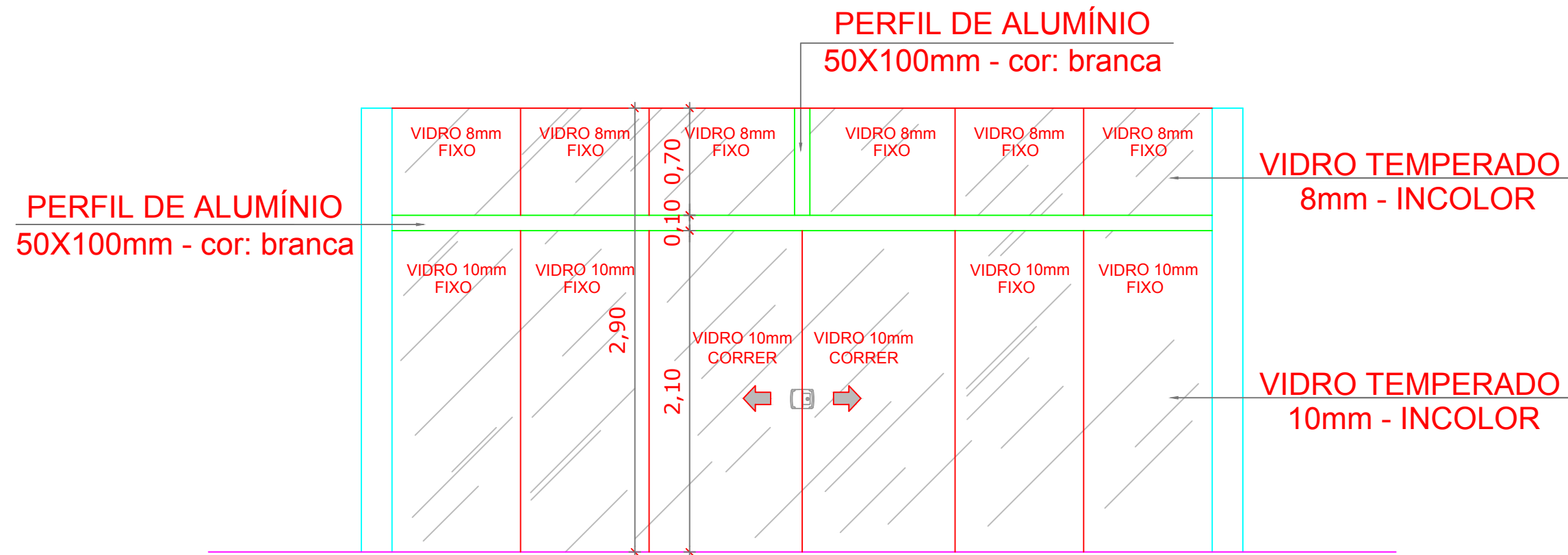
VISTA 2 ESC 1/50
