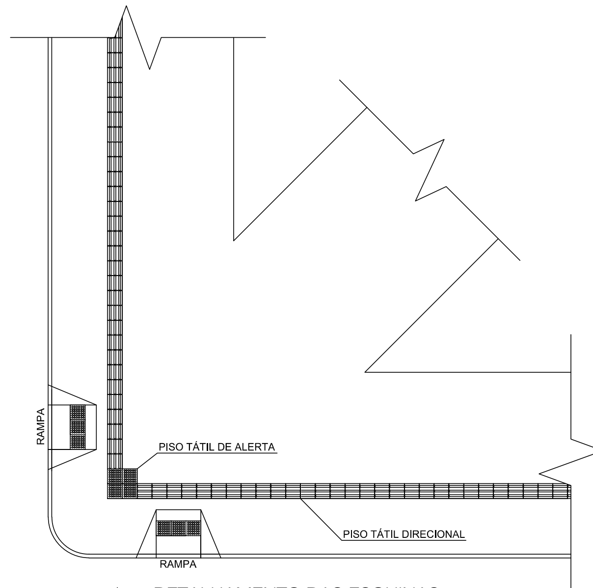
— ARQ DETALHAMENTO DAS ESQUINAS ESC: 1/100
