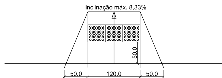
— ARQ DETALHAMENTO DAS RAMPAS ESC: 1/50
