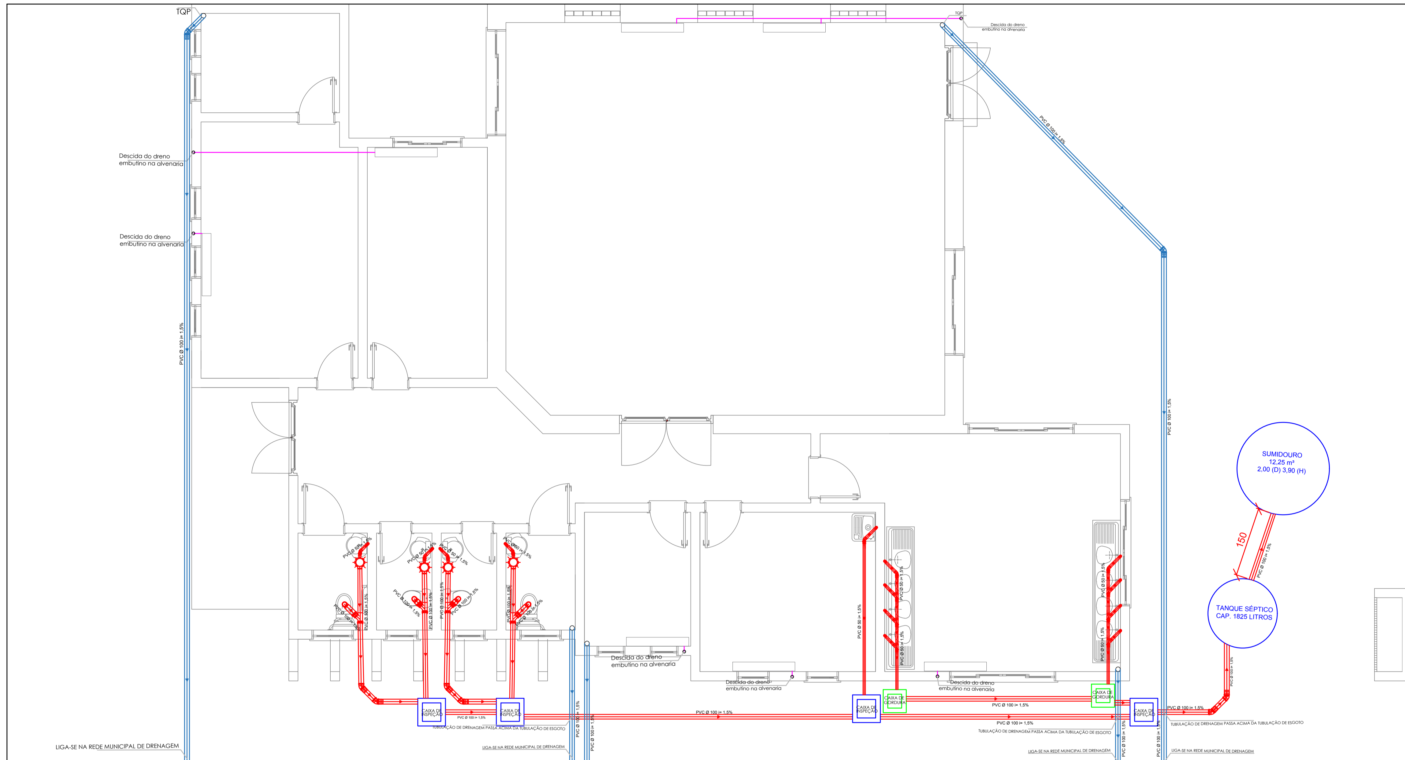
ENG INSTALAÇÕES SANITÁRIAS E PLUVIAIS ESCALA - 1/50
