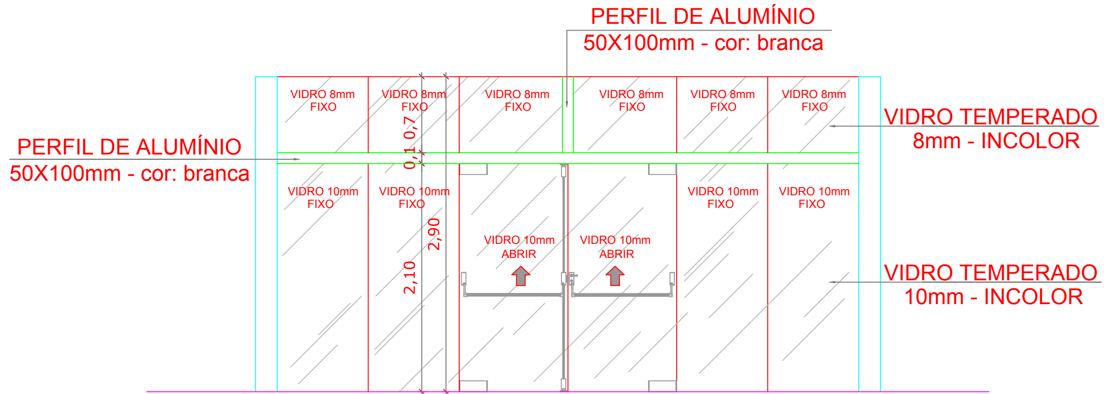
VISTA 1 ESC 1/50
