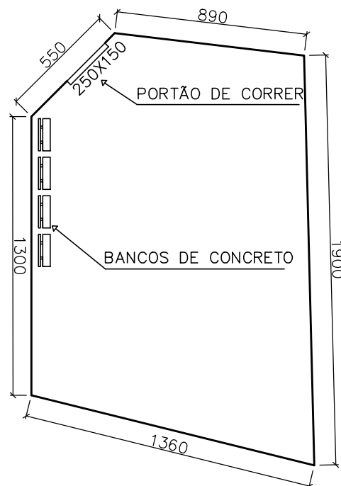
— ARQ PARQUINHO INFANTIL ESC: 1/250 COMPRIMENTO CERCADO: 60,00m
