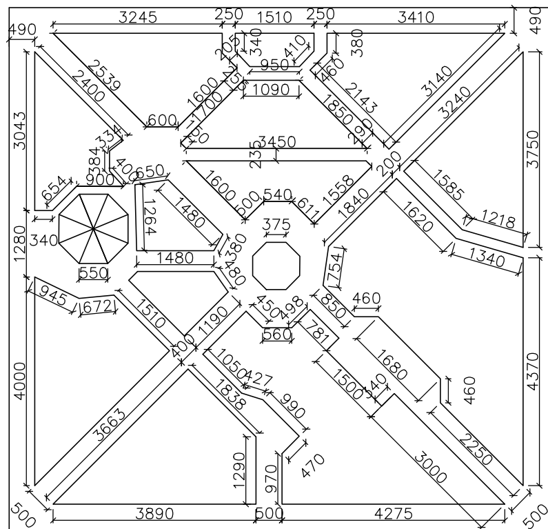
— ARQ PLANTA BAIXA ESC: 1/1000 Área total do piso: 4.298,14m 2
